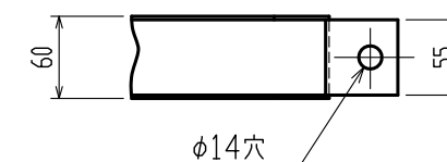
台座/脚部分詳細(S=1/6)
