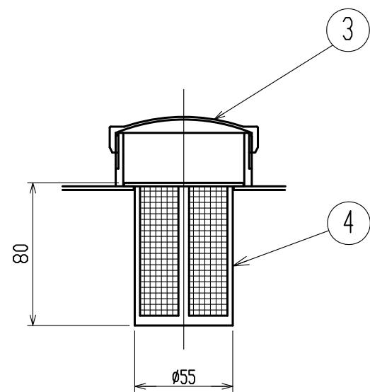
給油口付近詳細(S=1/3)
