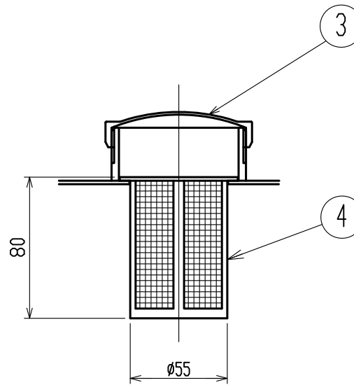
給油口付近詳細(S=1/3)
