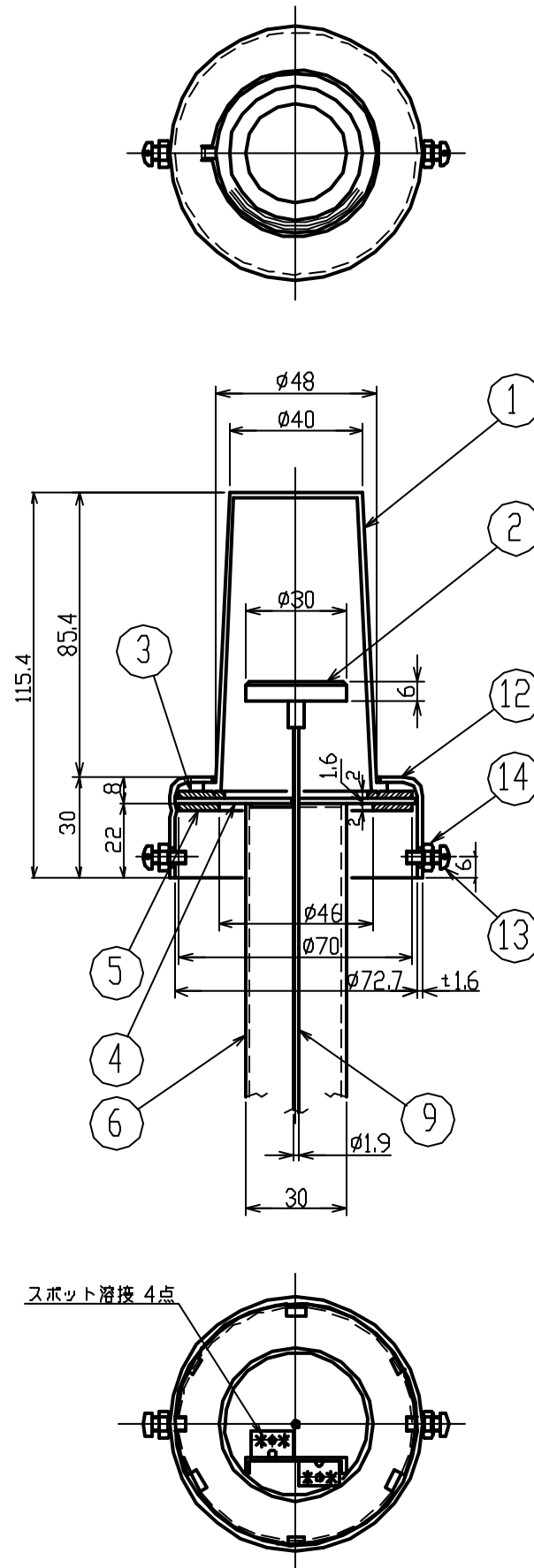
詳細図 (S=1/2)
