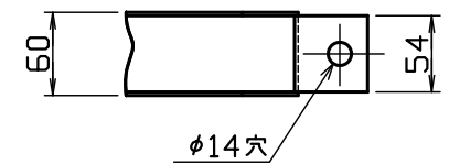
台座/脚部分詳細(S=1/6)
